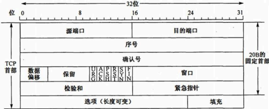
题 47-b 图 TCP 段头结构
